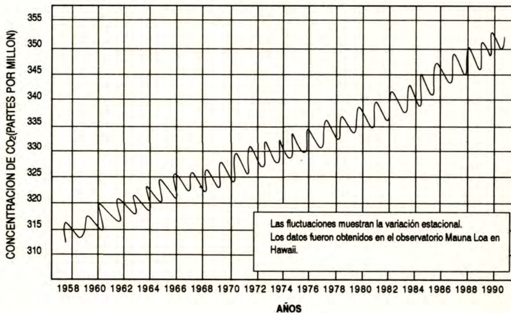
AUMENTO DE BIXIDO DE CARBONO (CO 2 ) EN LA ATMOSFERA
